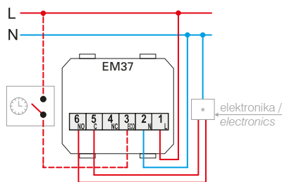
bojler, toplinska crpka, plamenik (upravljački unos T1/T2) / boiler, heat pump, burner (control input T1/T2)
