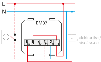
circulacijska crpka, plamenik (direktno spajanje) termoelektrični pogon / circulation pump, burner (direct connection) thermoelectric drive
