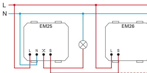
(2) Trožični trožični spoj three-wire connection
